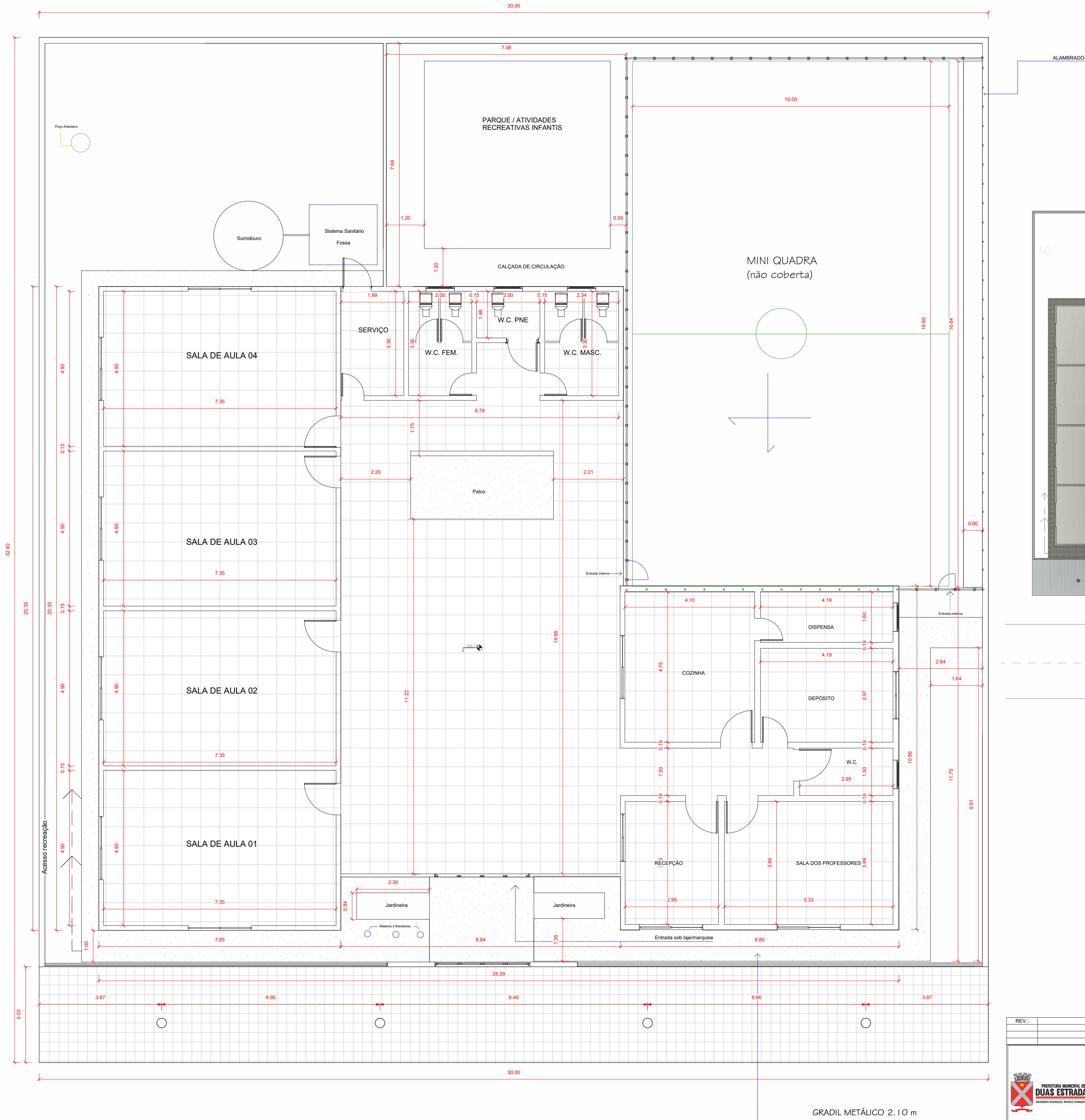
① PLANTA BAIXA TÉCNICA - TÉRREO 1 : 75
